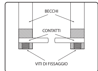
Installazione contatti
