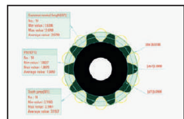
QUOTATURA AUTOMATICA
